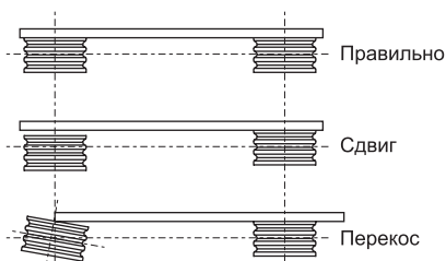
Рисунок 47. Выверка валов.
